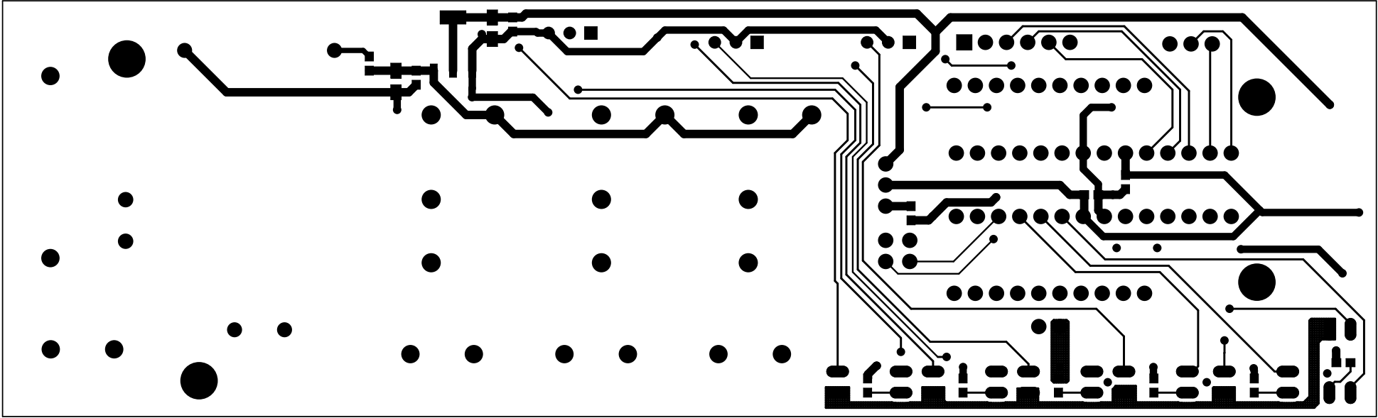
BOTTOM LAYER
